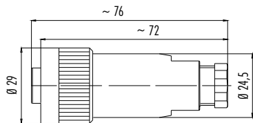
Maßzeichnung / Drawing
